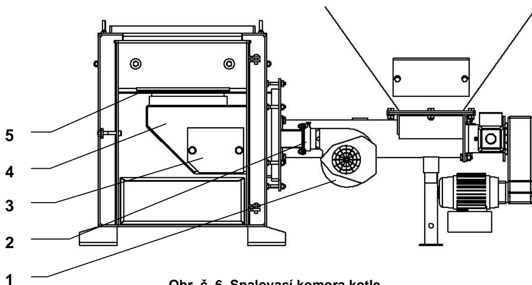
Obr. č. 6 Spalovací komora kotle
