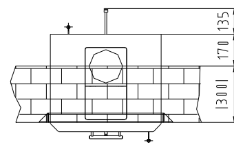
POHLED P
