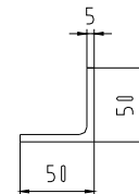
Průřez rámu
