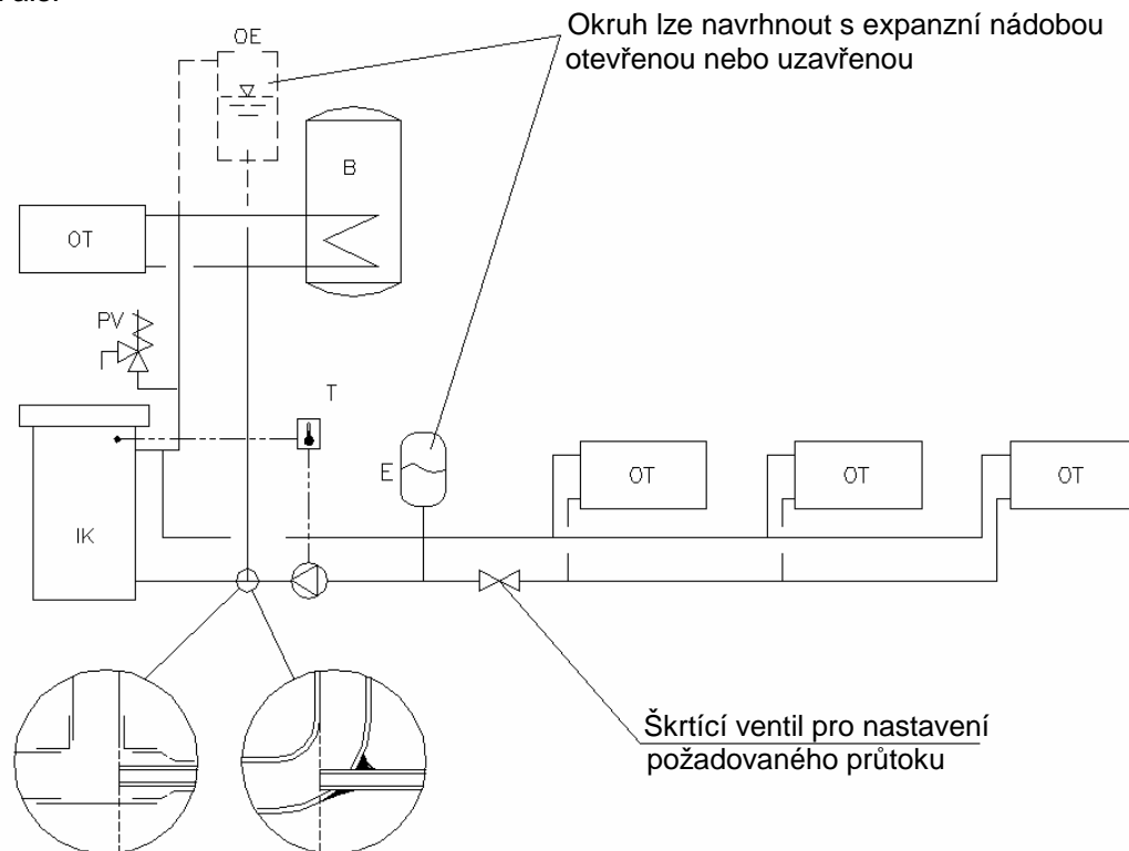
PŘÍKLADY PŘIHOJENÍ
