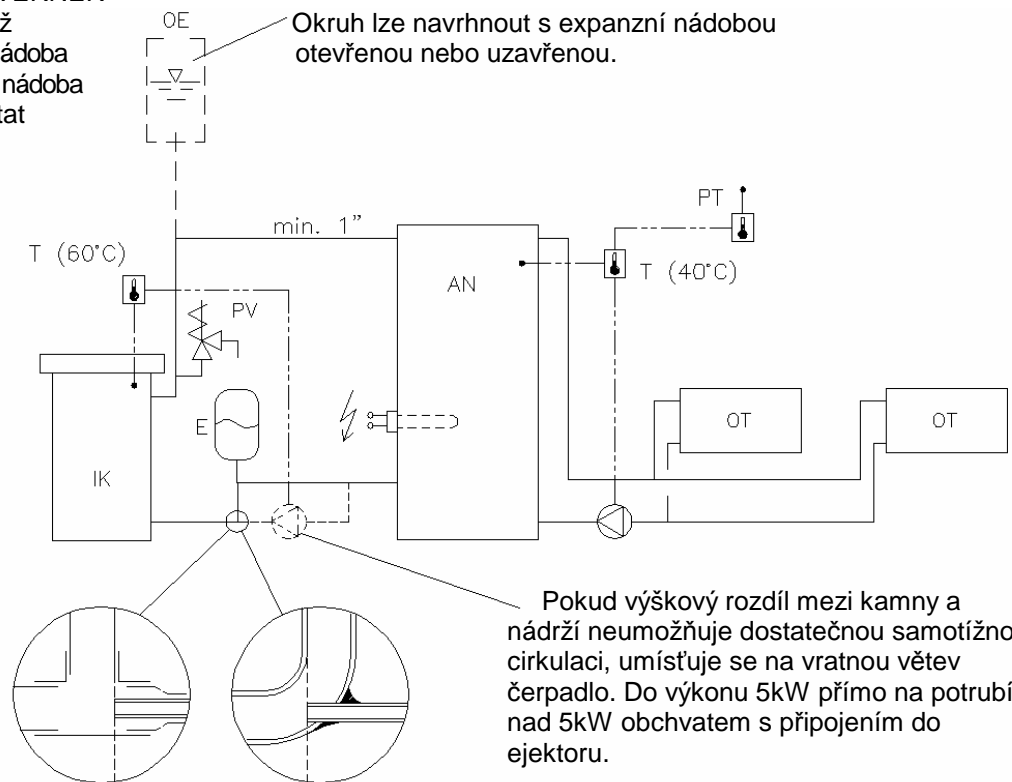
PŘÍKLADY PŘIPOJENÍ
