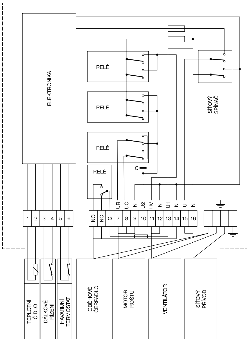
Obr. 2 Svorkové schéma regulátorů ADEX a SL-3.2
